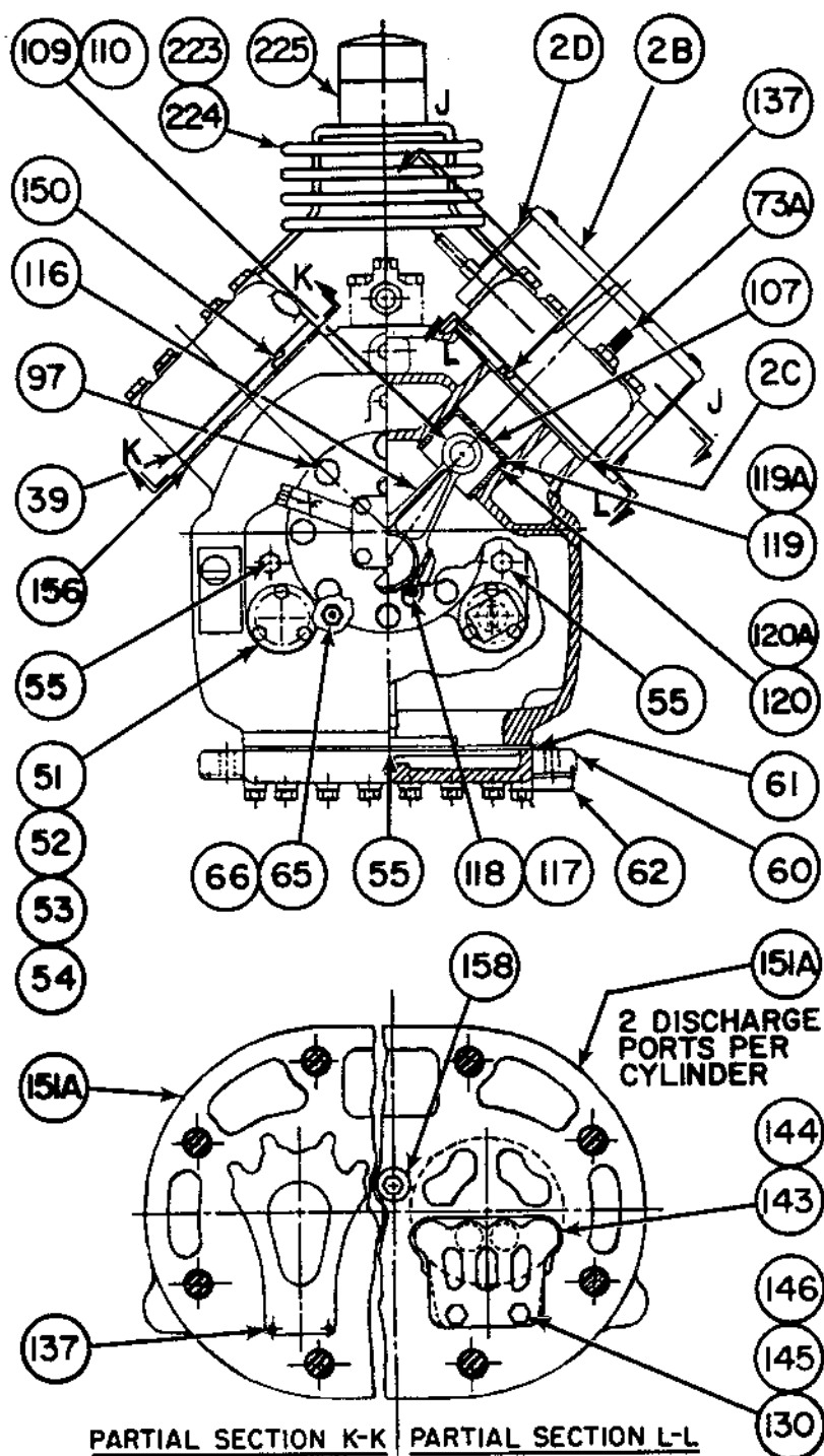
06E/06R/EY (4 CYLINDER)
